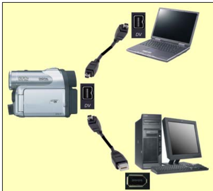
Conexión IEEE 1394 para videocámara digital
